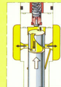
Förderende
