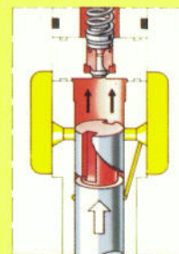
Förderbeginn
