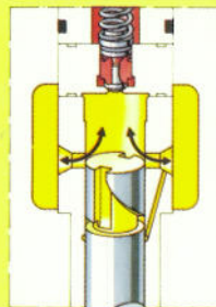
Unterer Totpunkt
