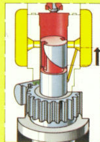
Vollförderung
