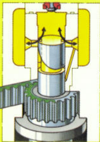
Nullförderung
