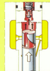
Förderung
