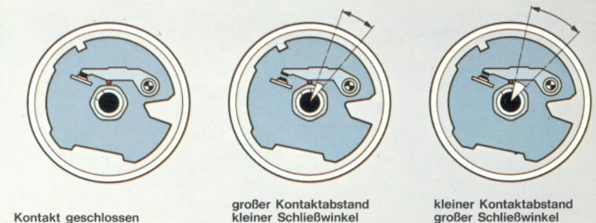
Unterbrecherkontakt
