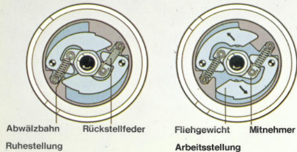
Fliehkraftversteller, abhängig von Drehzahl
