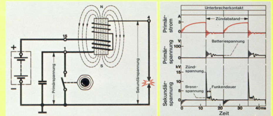
Unterbrecherkontakt
