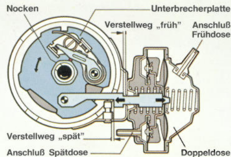
Unterdruckversteller in Richtung früh und spät
