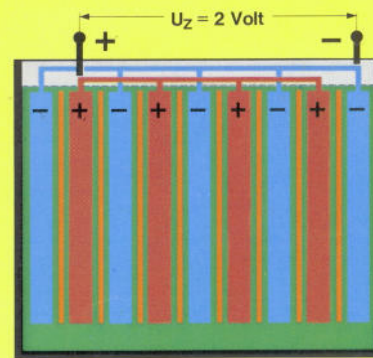
Zelle
