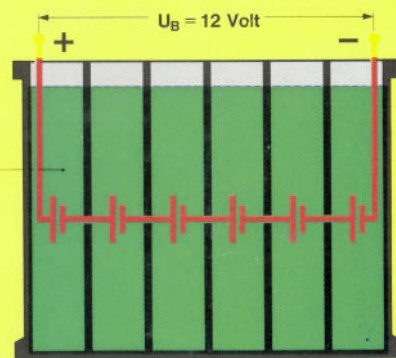
Batterie
